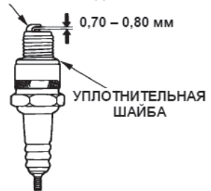
БОКОВОЙ ЭЛЕКТРОД
